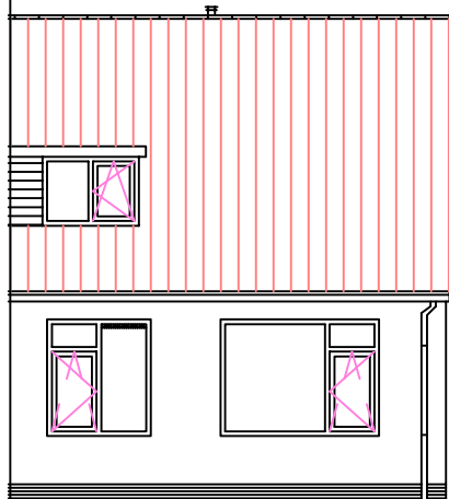
Voorgevel
