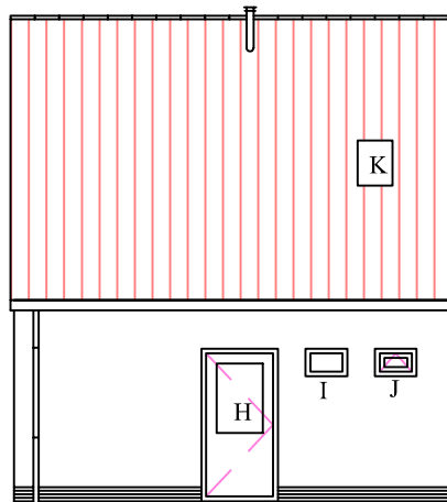
Achtergevel
