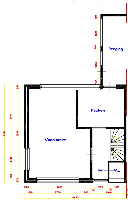
Begane Grond
