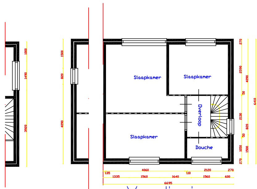
Verdieping
