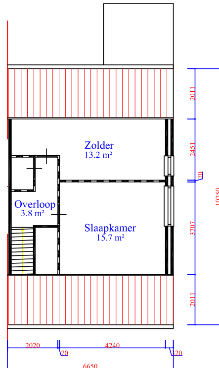
Verdieping
