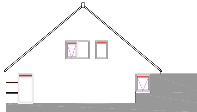
R.Zijgevel
