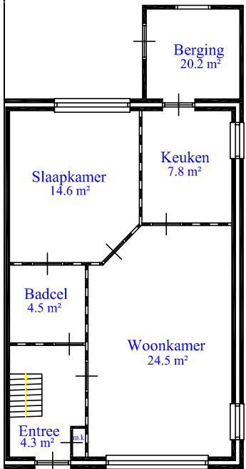
Begane Grond
